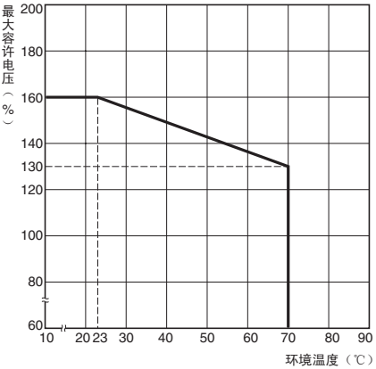
环境温度与最大容许电压
