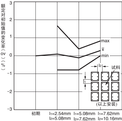
磁气干扰 (继电器相互)
