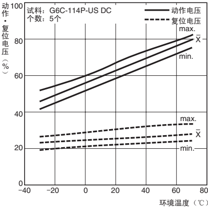
环境温度与动作、复位电压
