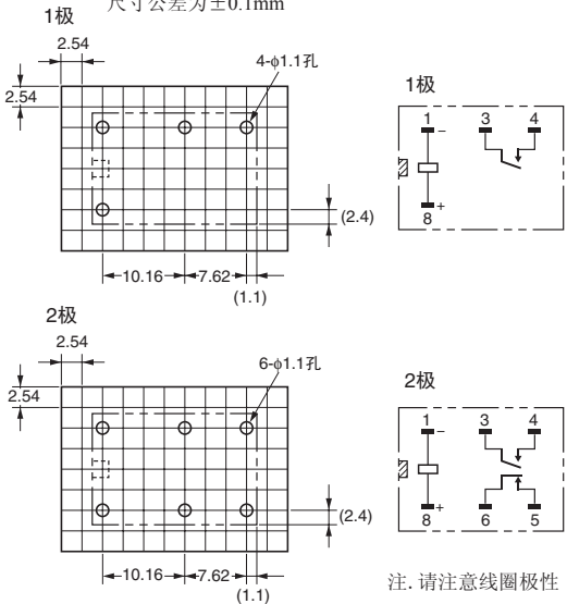
端子配置/内部连接图 (BOTTOM VIEW)
